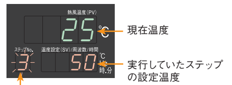
プログラム運転でない熱風運転時の表示
