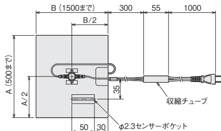
● 寸法図
