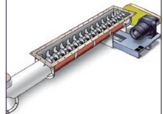
土壌滅菌用 (スクリュコンベア)
