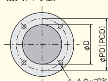
吸入口寸法
