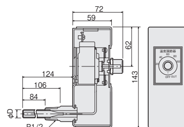
● EAC-3LT, 4LT 寸法図
