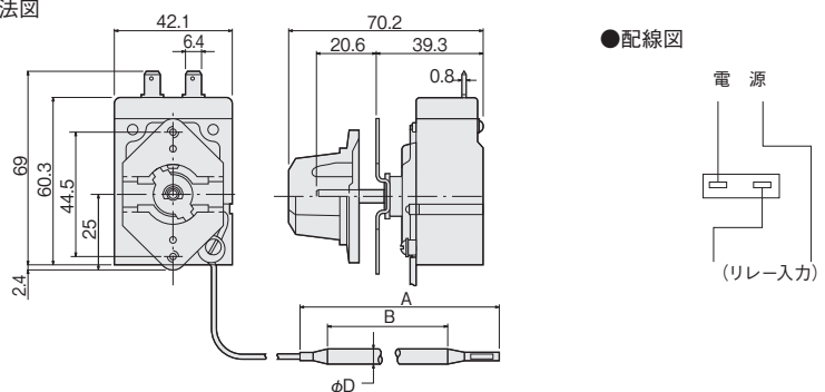
● 寸法図
