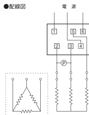
●配線図
