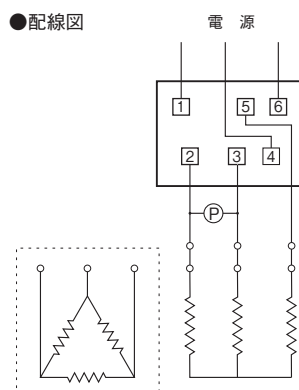
●配線図
