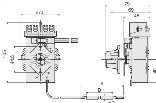
●寸法図
