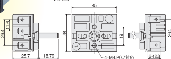
寸法図
