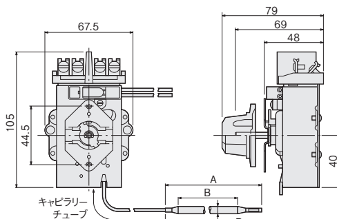
●寸法図
