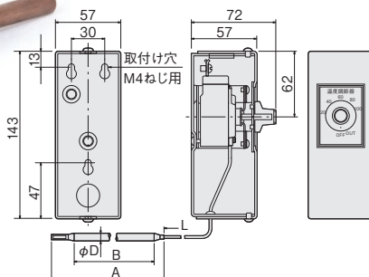
● EAC 寸法図
