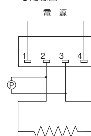
●配線図
