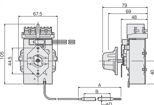
●寸法図
