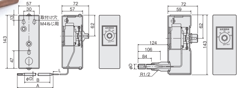
● EAC 寸法図
