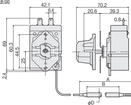
● 寸法図
