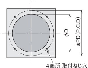
吸入口ボックス寸法
